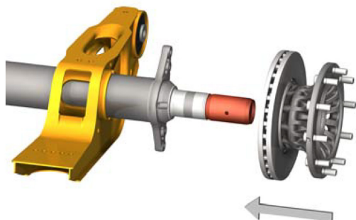
Abb. 2: Montage bei scheibengebremsten Achsen
