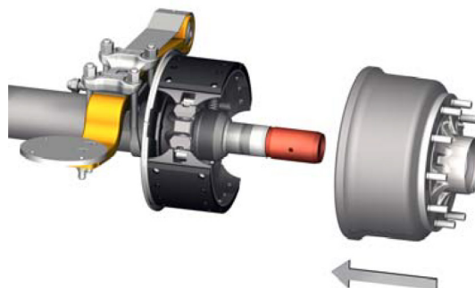
Abb. 3: Montage bei trommelgebremsten Achsen
